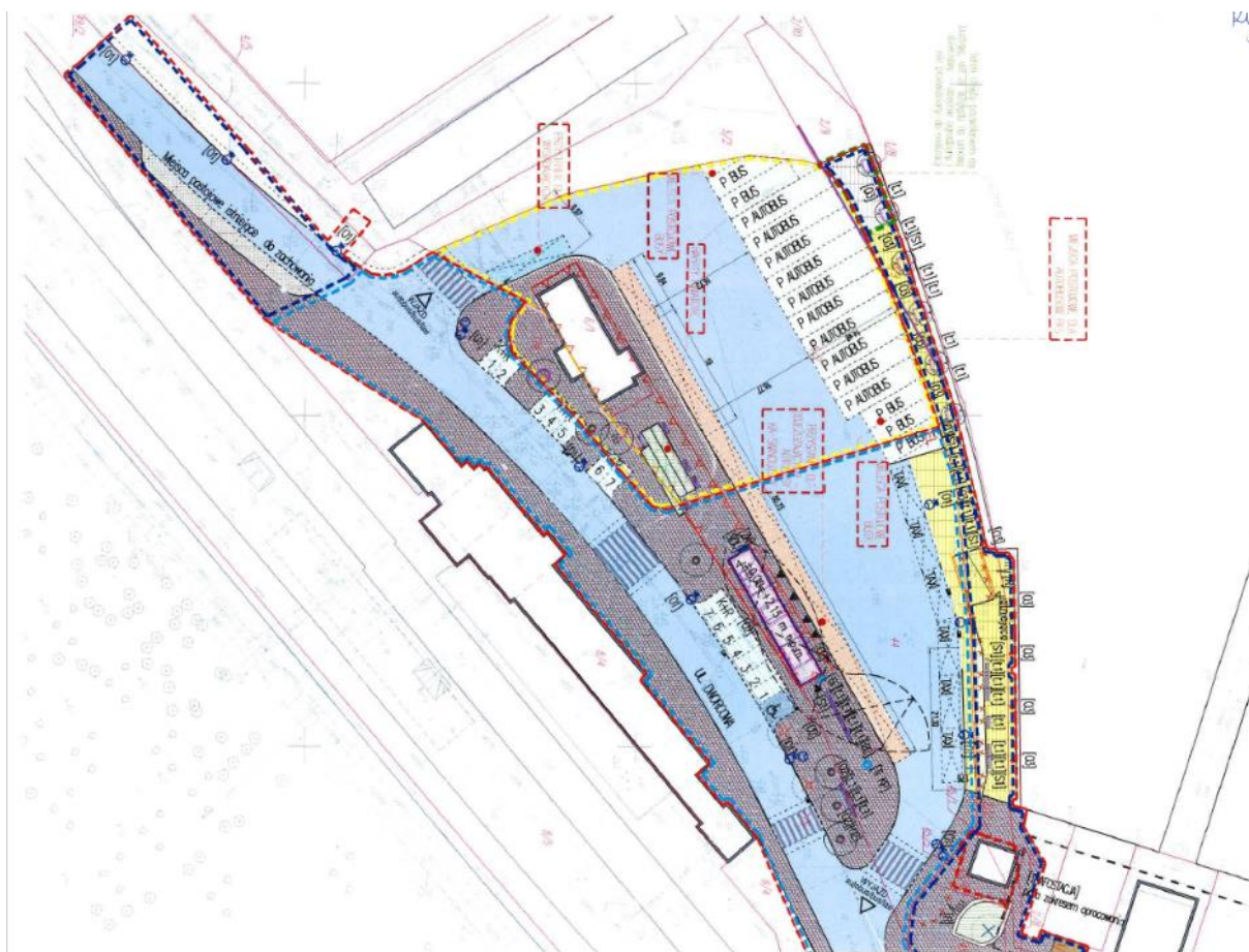
Rysunek 11 Koncepcja zmian w wyglądzie placu przy dworcu kolejowym
