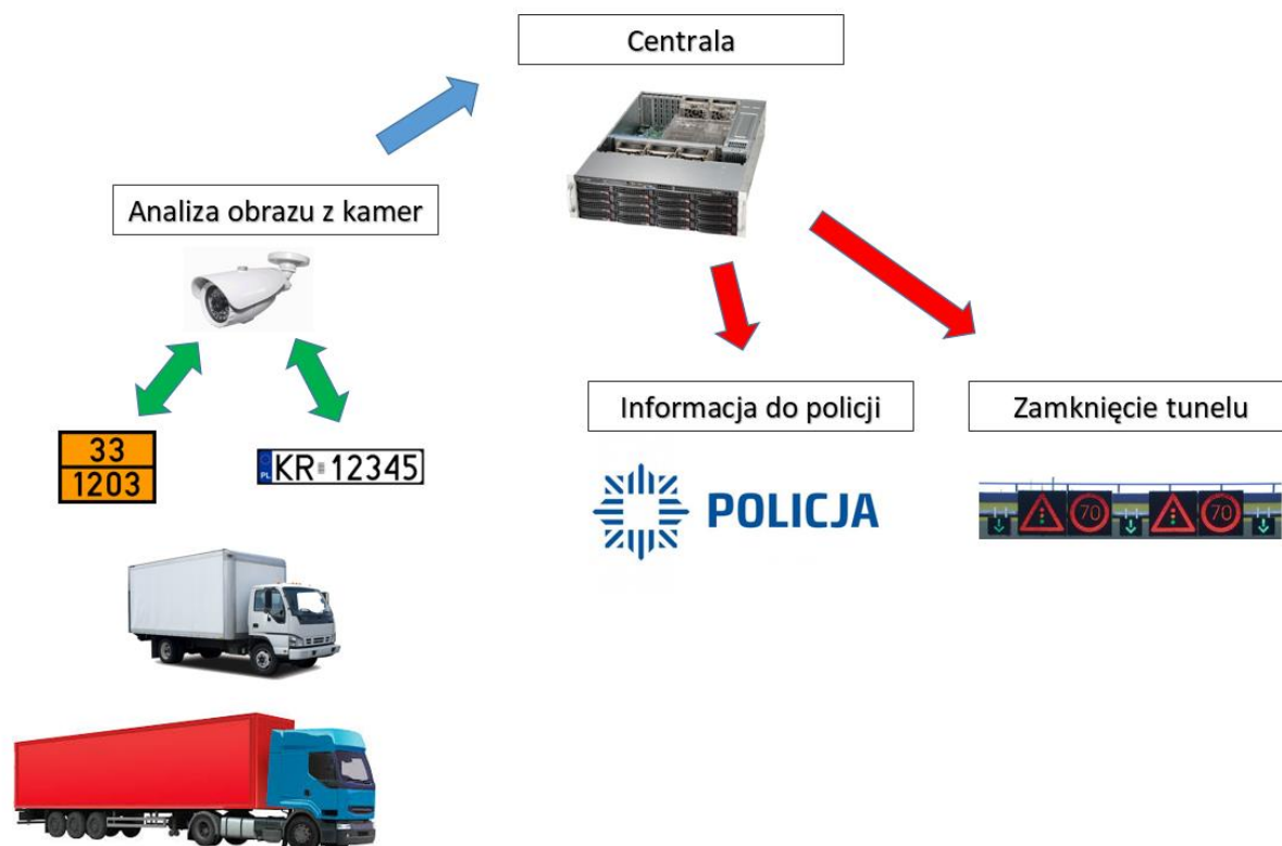
Rysunek 38 Przykładowy schemat działania systemu wykrywającego łamanie zakazu wjazdu do tunelu
