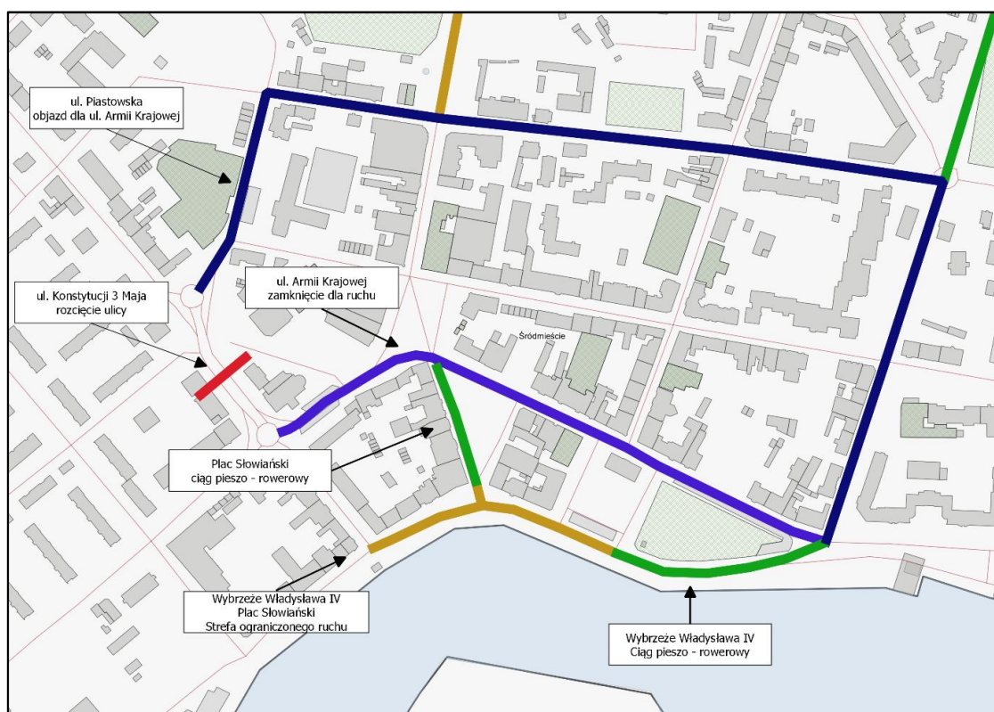
Rysunek 27 Propozycja zmian w organizacji ruchu drogowego w Świnoujściu – scenariusz silniejszy
