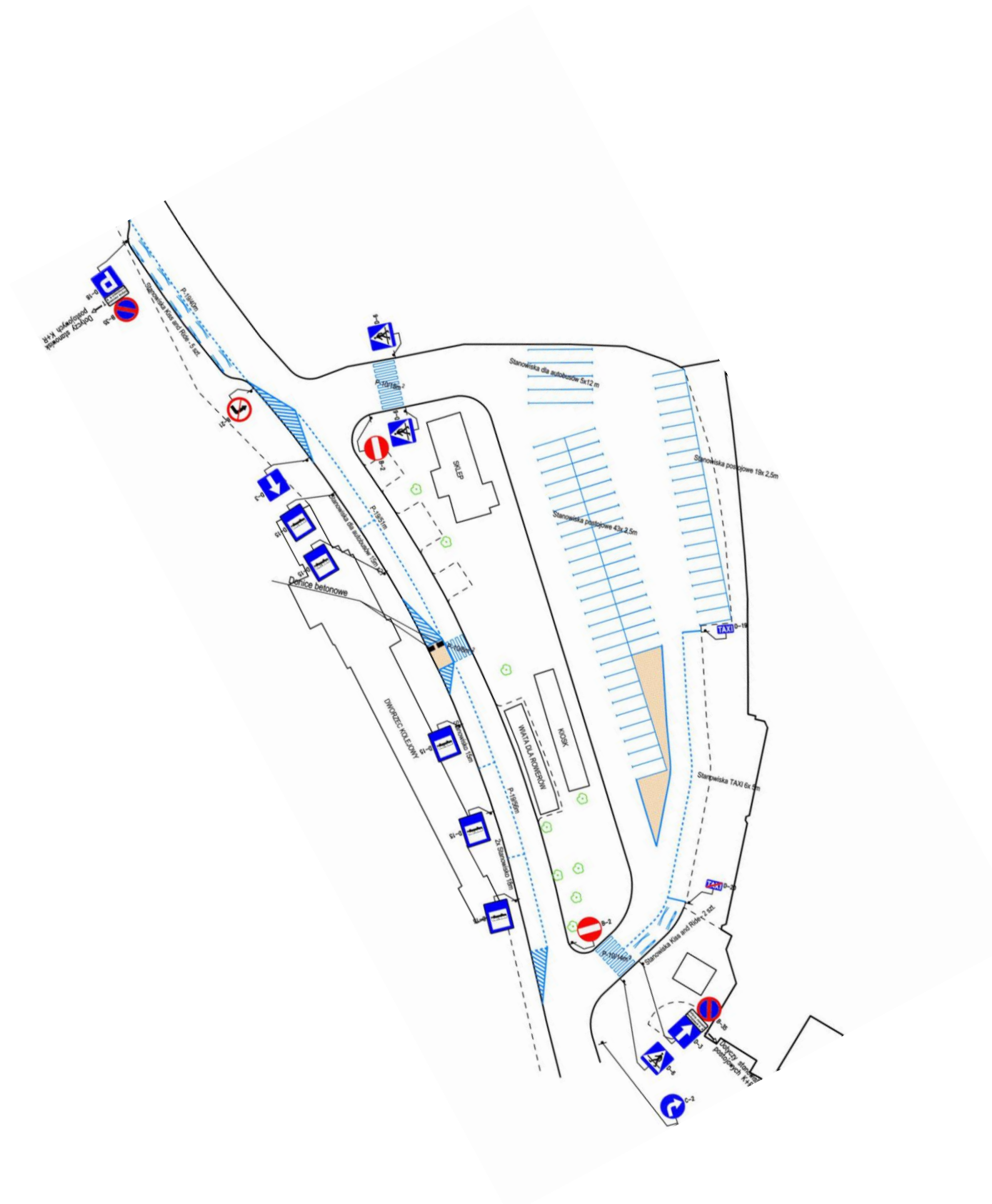
Rysunek 12 Propozycja weryfikacji zmian w organizacji ruchu na placu przy dworcu kolejowym
