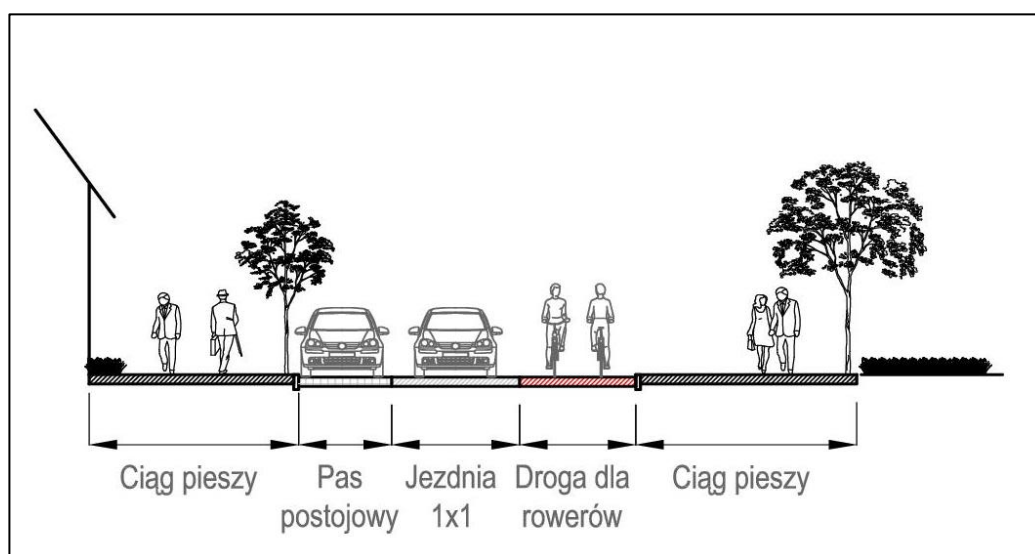
Rysunek 23 Przekrój poprzeczny na ul. Matejki – propozycja zmian
