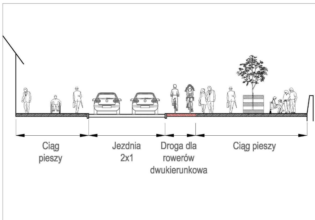
Rysunek 26 Przekrój poprzeczny na Wybrzeżu Władysława IV – propozycja zmian wariant II
