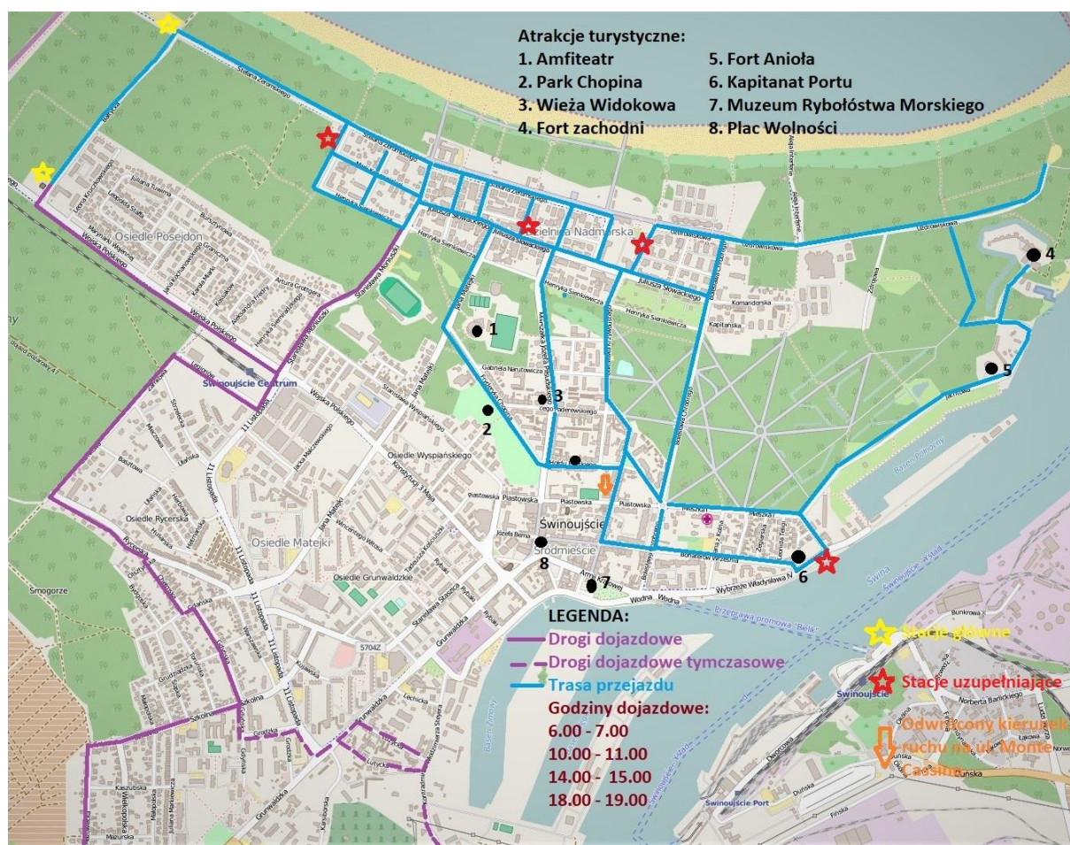
Rysunek 13 Trasy kursowania pojazdów wolnobieżnych
