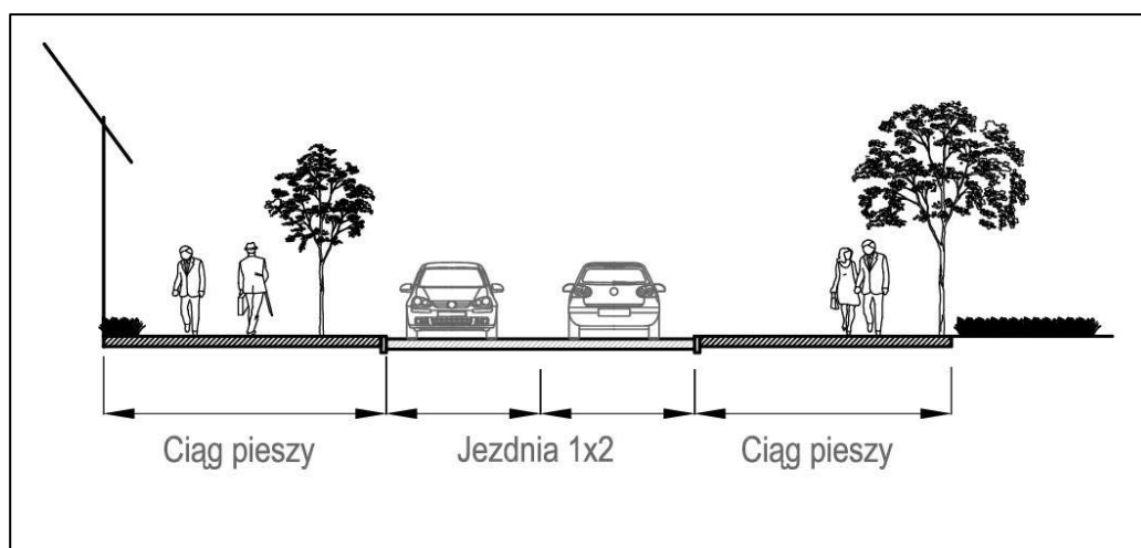
Rysunek 22 Przekrój poprzeczny na ul. Matejki – stan obecny
