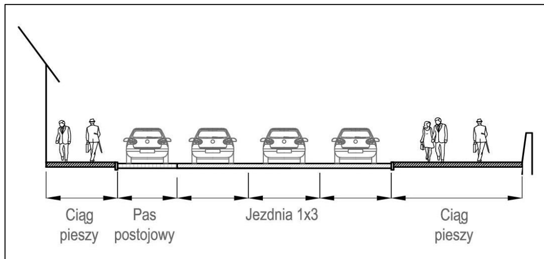
Rysunek 24 Przekrój poprzeczny na Wybrzeżu Władysława IV – stan obecny
