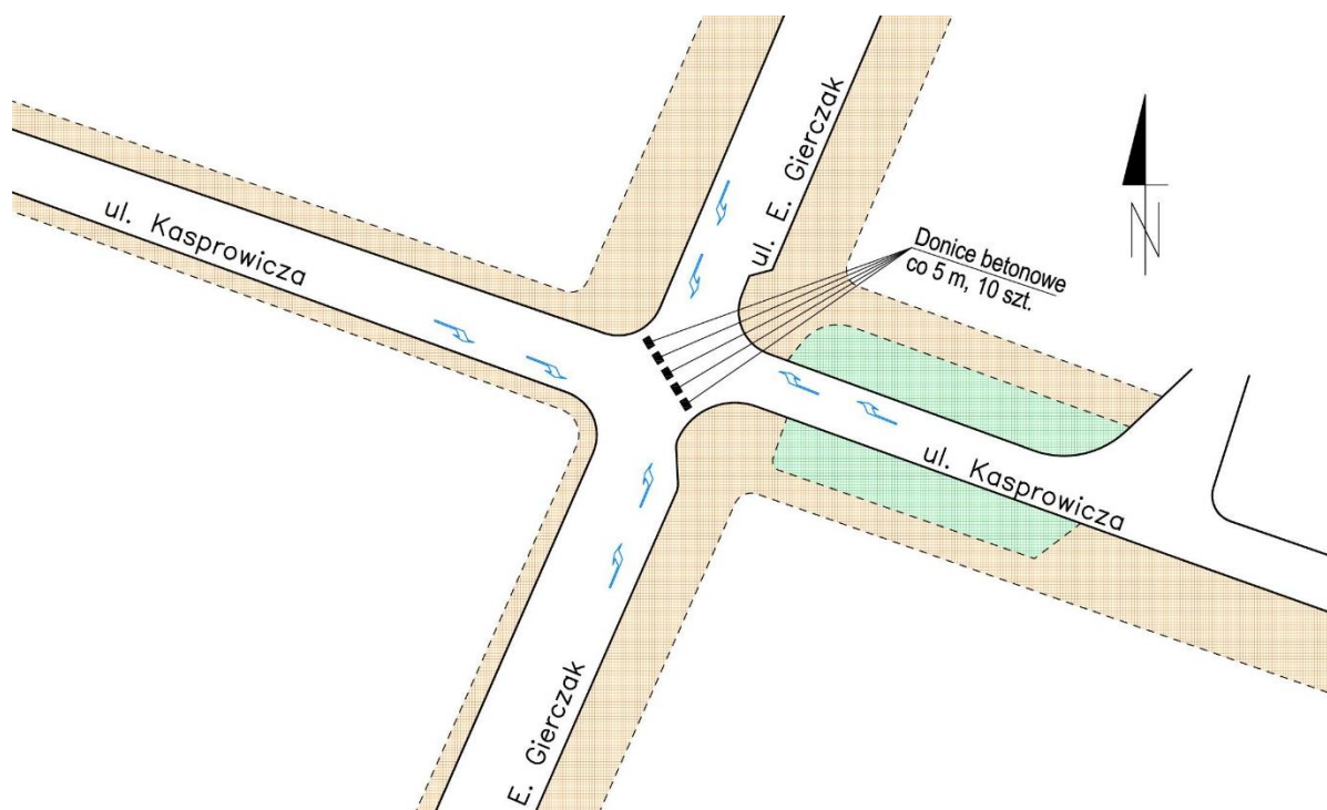
Rysunek 21 Propozycja zmiany w organizacji ruchu na skrzyżowaniu ulicy Emilii Gierczak i Kasprowicz
