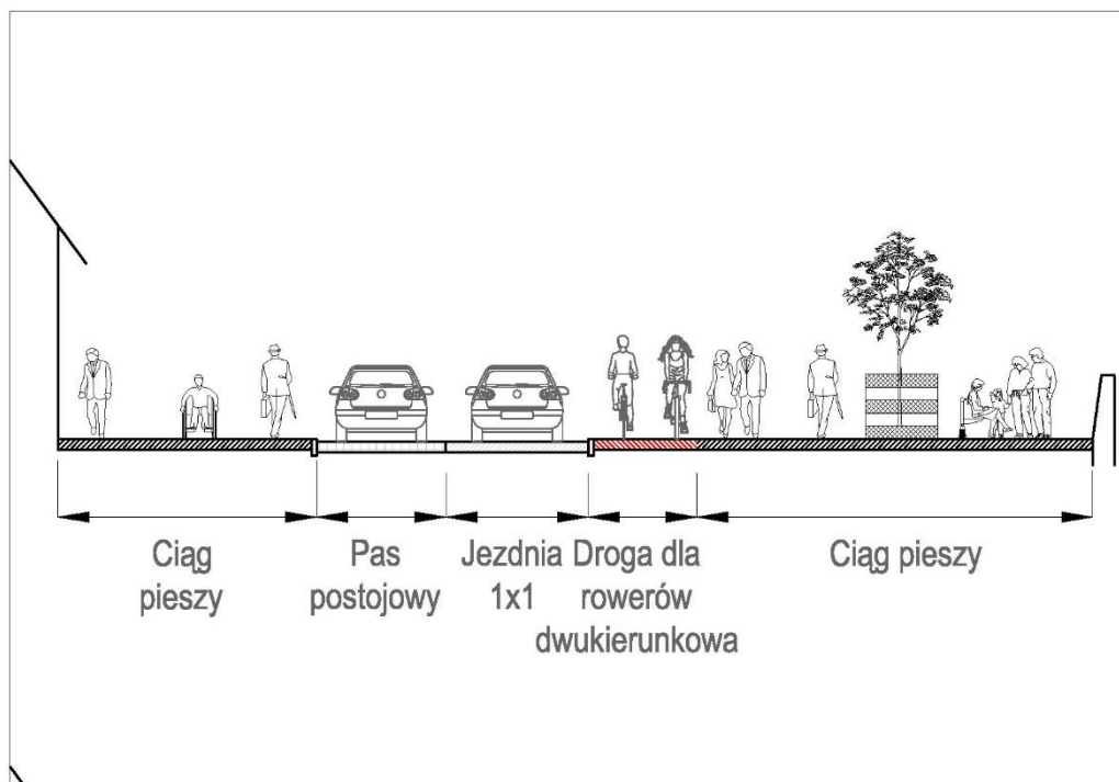
Rysunek 25 Przekrój poprzeczny na Wybrzeżu Władysława IV – propozycja zmian wariant I
